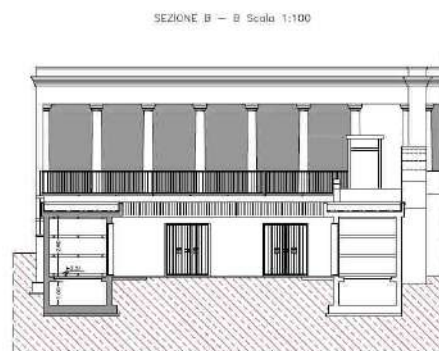
Prospetto
