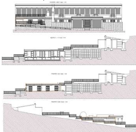
Sezioni - Prospetti
